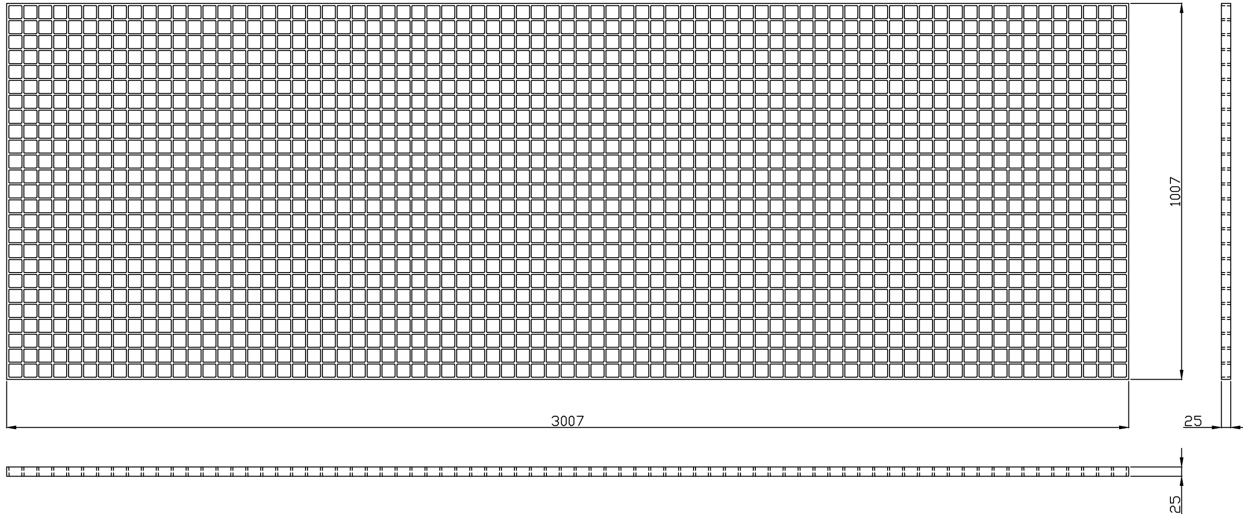
IバープレートG10型25H 定尺図 (FRP製グレーチング25H)
