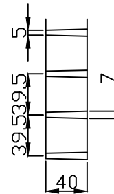
Iバーグレーティング型マスメ詳細図
