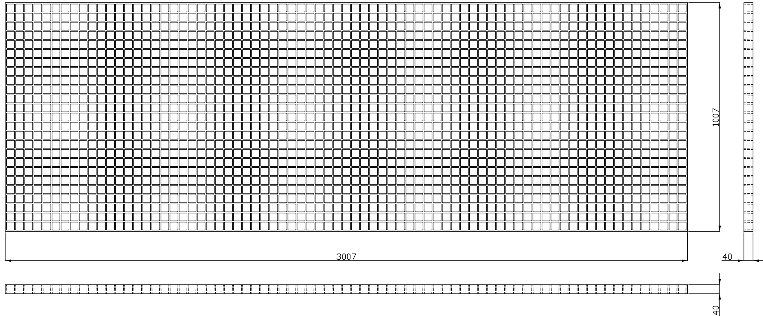
Iバー-プレートG10型40H 定尺図 (FRP製グレーチング40H)
