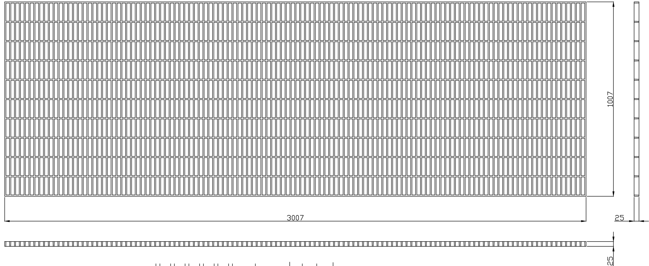
Iバーグレーティング5型25H 定尺図 (FRP製グレーティング25H)
