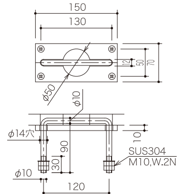
【CP用落とし込み取手】
